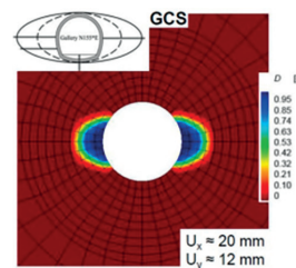
Calcul de l'endommagement autour d'une galerie, pour deux orientations différentes.
