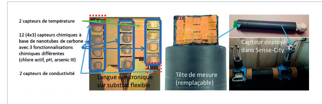
Tests dans l'équipement de recherche Sense-City d'un capteur multi-paramètres à nanotubes de carbone pour la qualité de l'eau. © Univ. Eiffel
