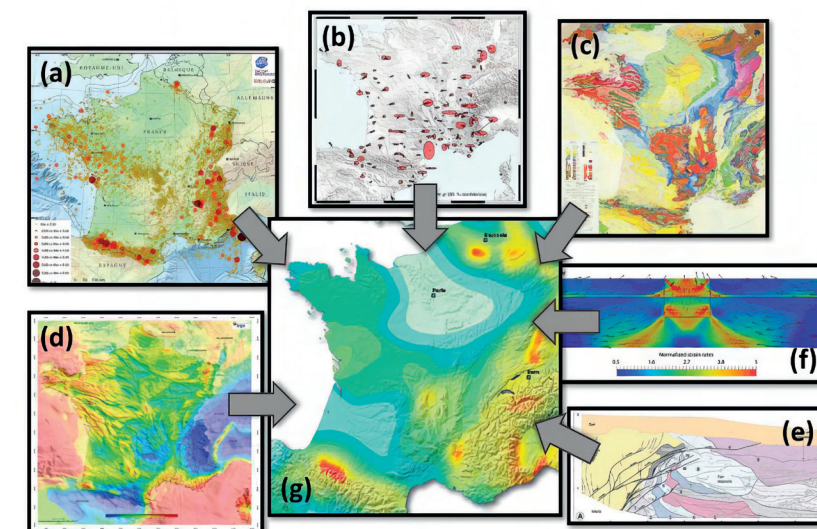
ALCESTE : un projet pour caractériser l'aléa sismique probabiliste en France métropolitaine
