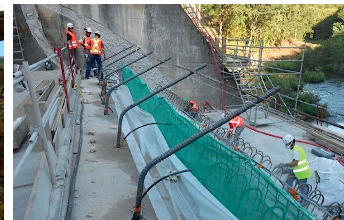
Des ancrages passifs installés dans le barrage. © Grégory Coubard
