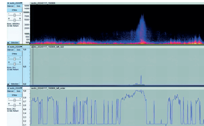
Détection des passages de TGV.
