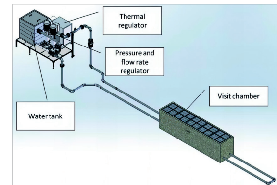
La boucle d'eau Sense-City. © Univ. Eiffel
